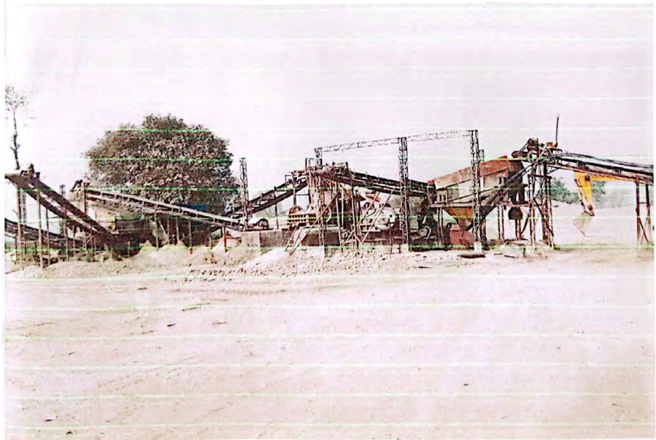
चित्र ५: मिनाक्षी एग्रीगेट इण्डस्ट्रिजमा जडान गरिएको बालुवा वाश प्लान्
